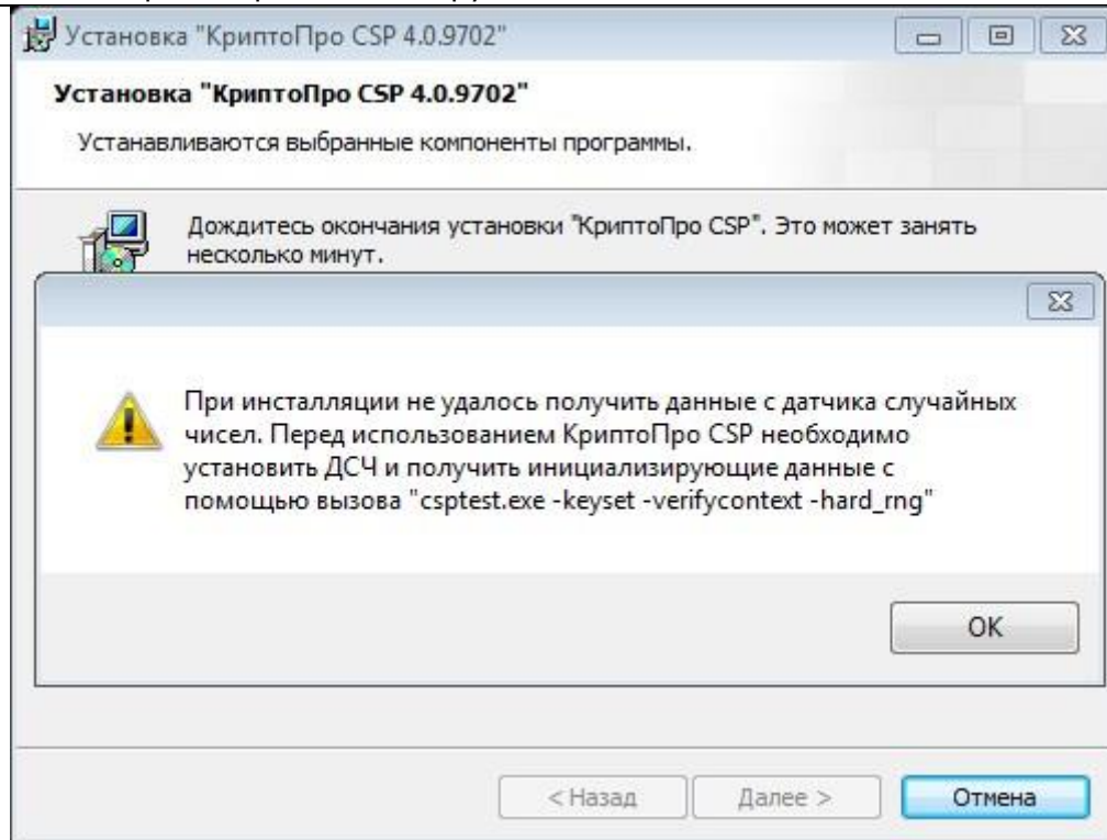
Рисунок 9. Окно ошибки получения данных с датчика случайных чисел при инсталляции СКЗИ.
