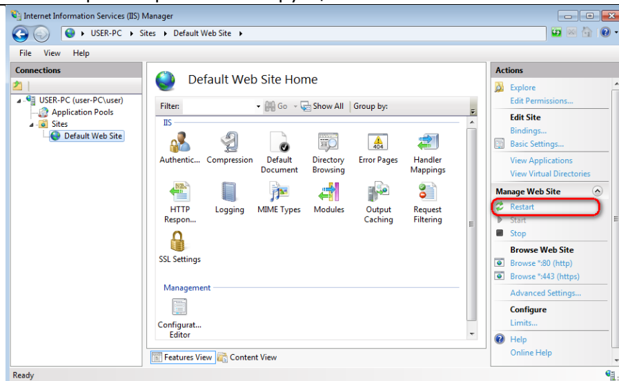
Рисунок 95. Перезапуск IIS
